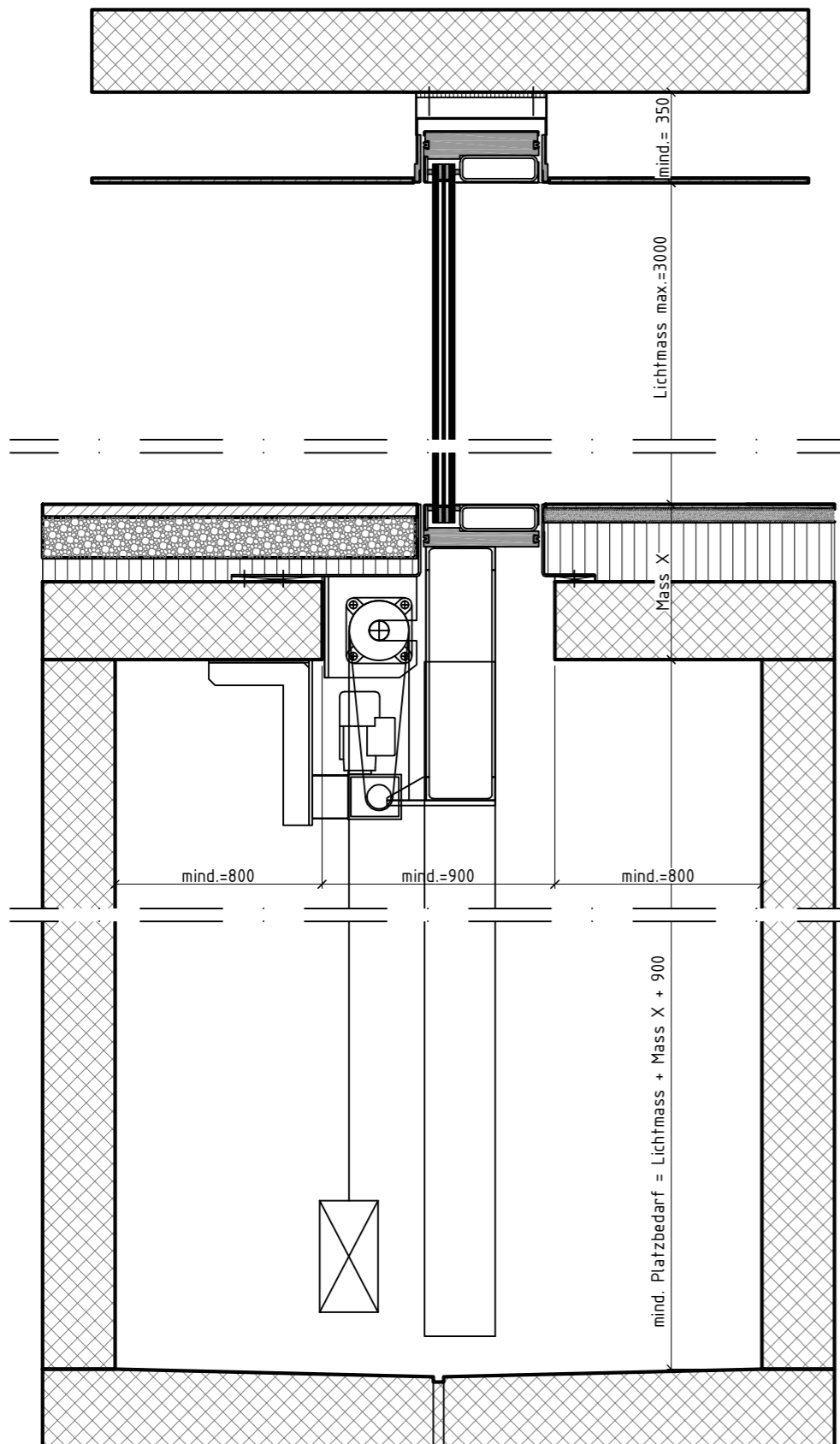
Schnitt A-A
