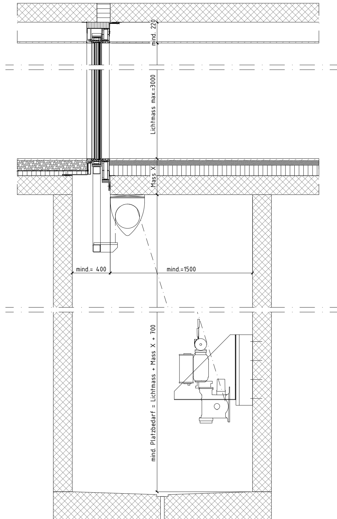
Schnitt A-A
