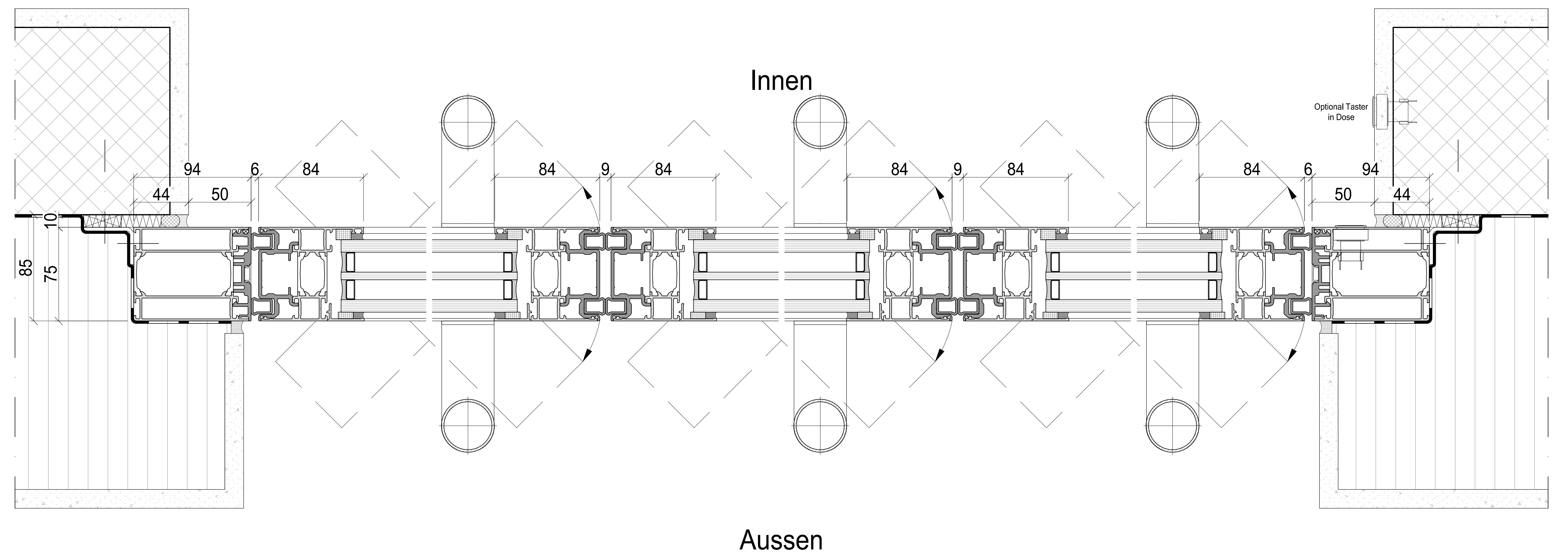
Schnitt C-C
